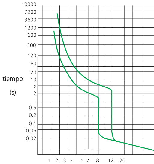
Curva característica para NM1-1250
