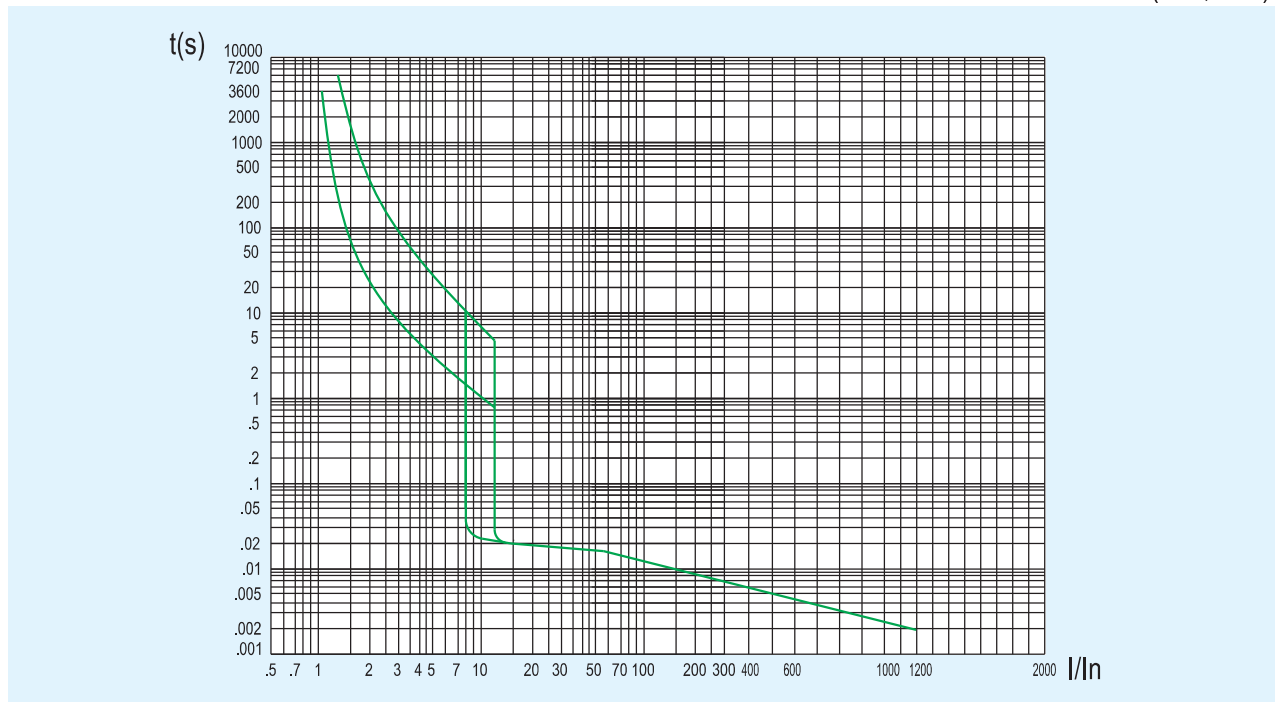
NM8-125(40A, 50A)
