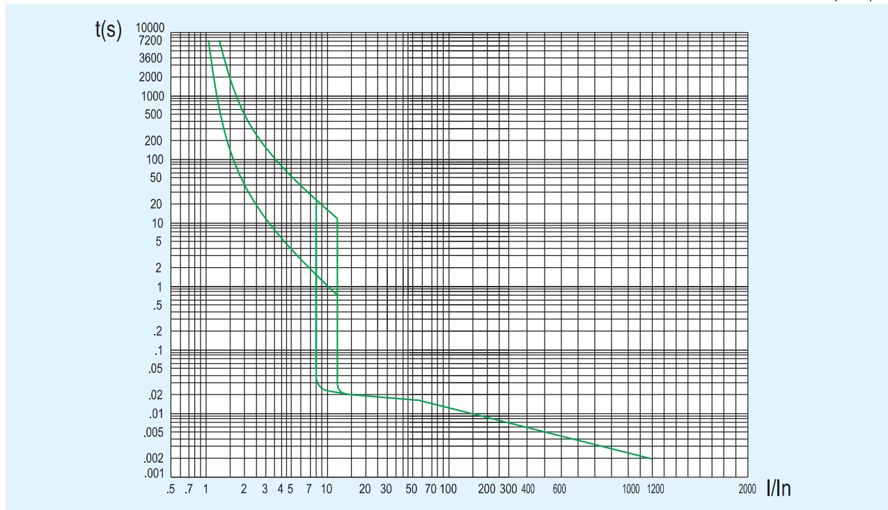
NM8-125(63A)
