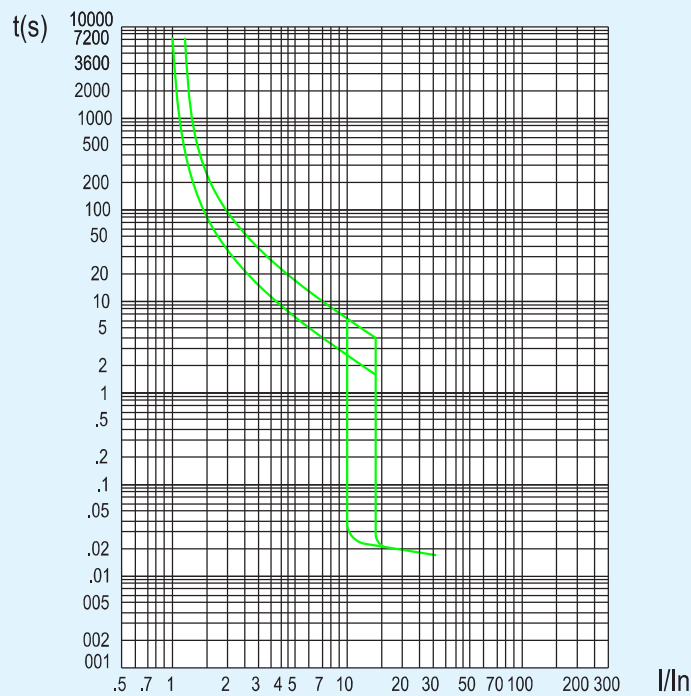
Protección de motores - NM8M-125, 250, 400, 630(16A~500A)
