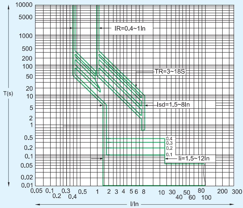
Protección de motores - NM8M-125, 250, 400, 630(16A~500A)
