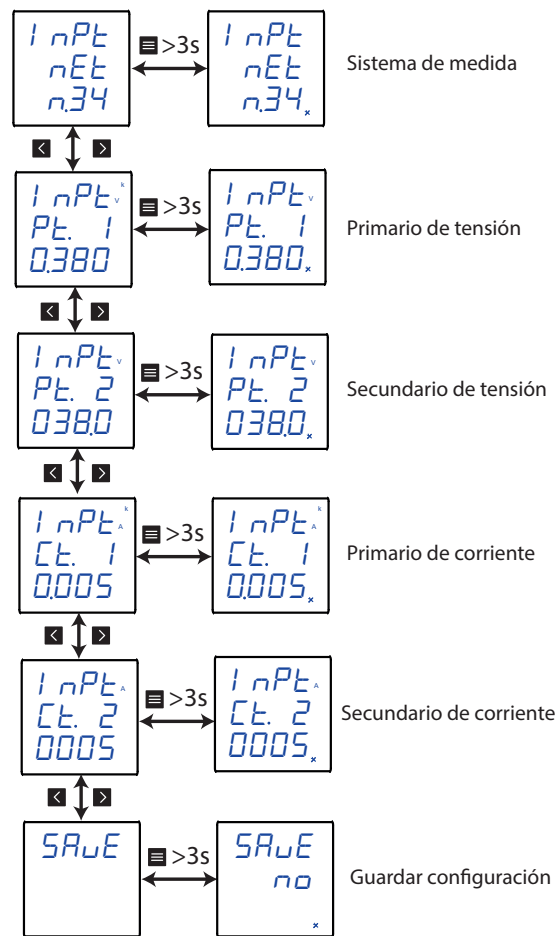
Figura 16: Menú de configuración de la entrada.
