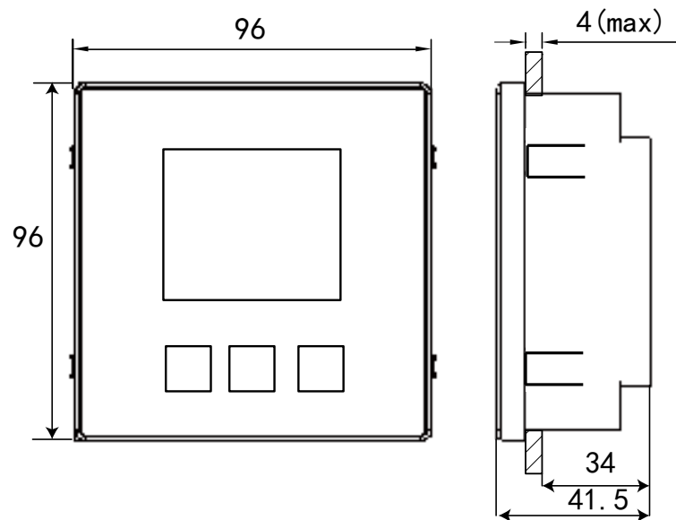
Figura 22: Dimensiones CVM-C4.
