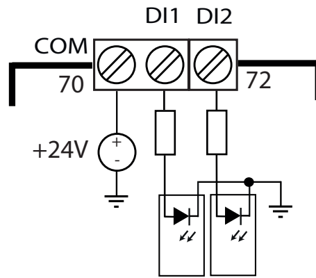
Figura 13: Entradas digitales.
