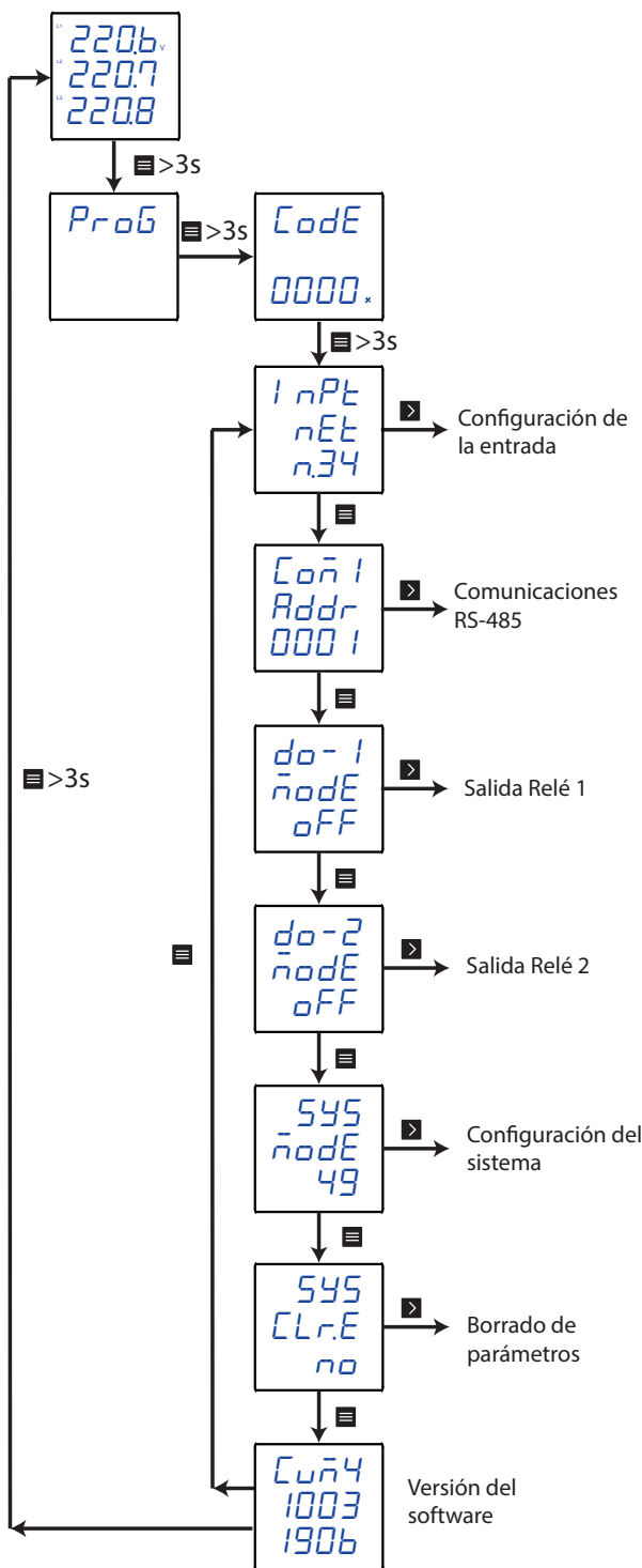
Figura 14: Menú de configuración CVM-C4.
