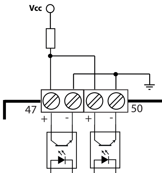
Figura 12: Salidas de pulsos de energía.
