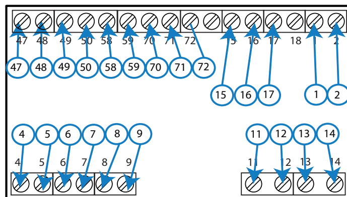
Figura 4: Bornes CVM-C4.
