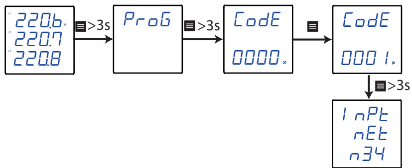
Figura 15: Acceso al menú de configuración en modo programación.
