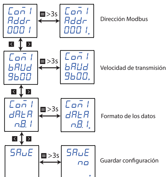
Figura 17: Menú de configuración de las comunicaciones RS-485.
