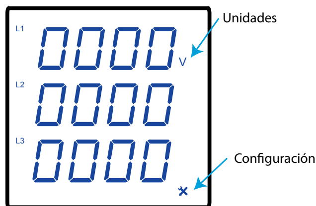
Figura 10: Display CVM-C4.
