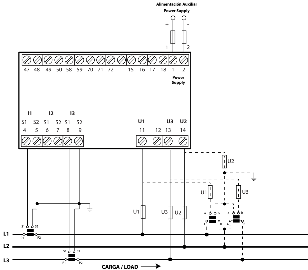
Figura 6: Medida de red trifásica con conexión a 3 hilos (Conexión 1).
