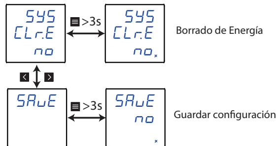
Figura 20: Menú de configuración del borrado de parámetros.
