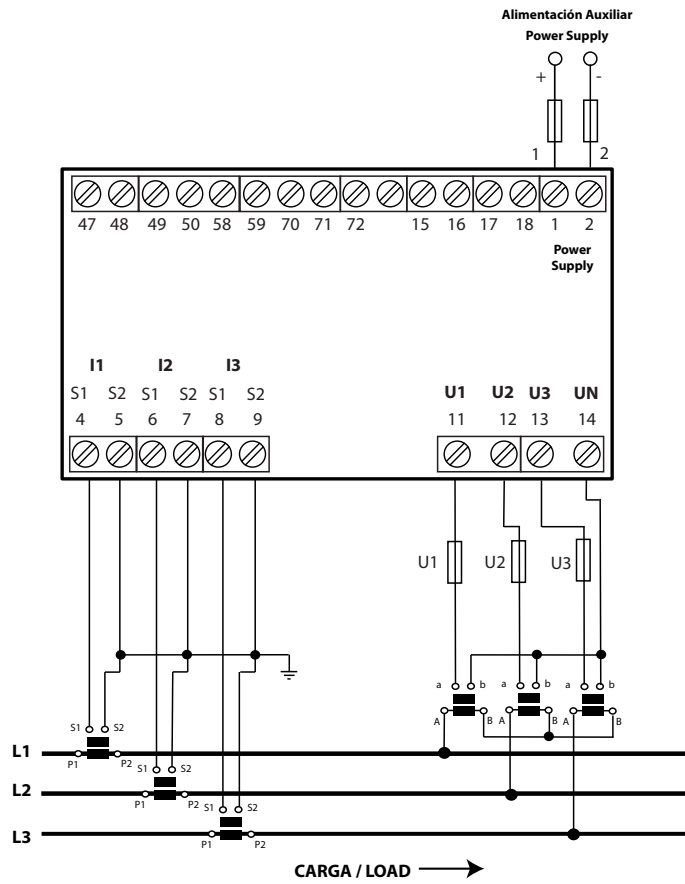
Figura 8: Medida de red trifásica con conexión a 3 hilos (Conexión 3).
