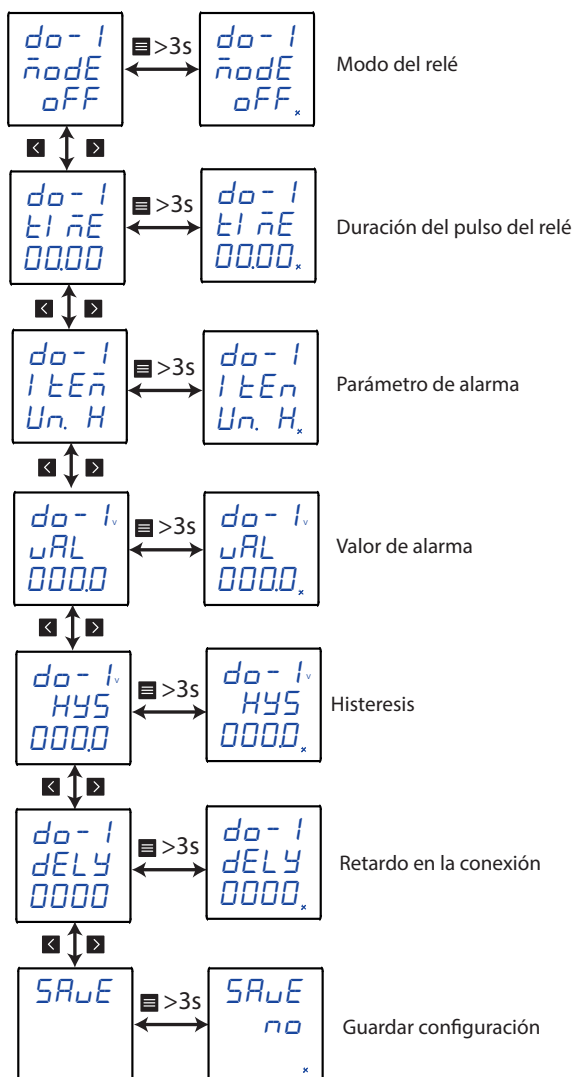
Figura 18: Menú de configuración de la salida de relé 1.
