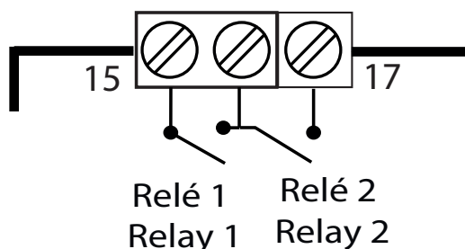
Figura 11: Salidas de relés.
