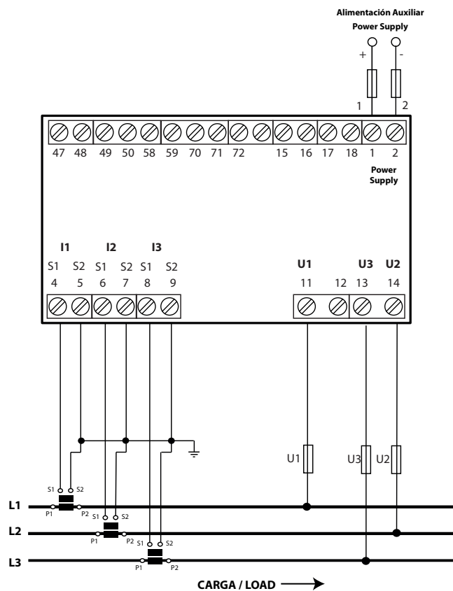
Figura 7: Medida de red trifásica con conexión a 3 hilos (Conexión 2).
